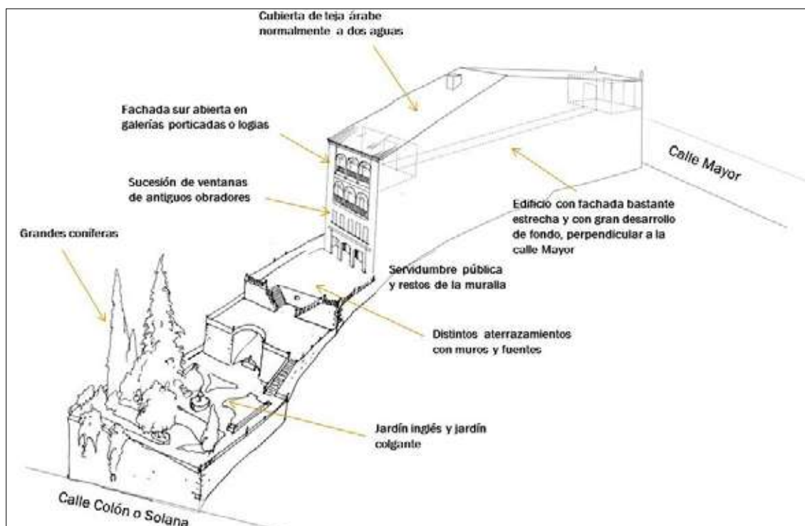
Plano de una casa burguesa en Béjar | ÓSCAR RIVADENEYRA
