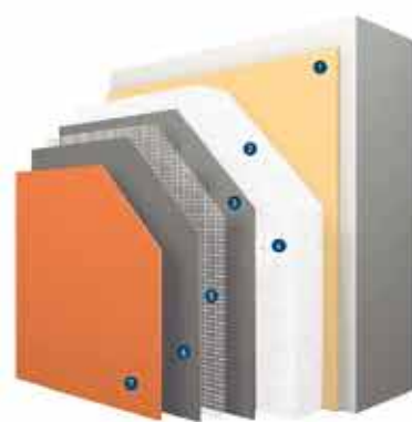
Figura 1. Configuración del sistema SATE.
